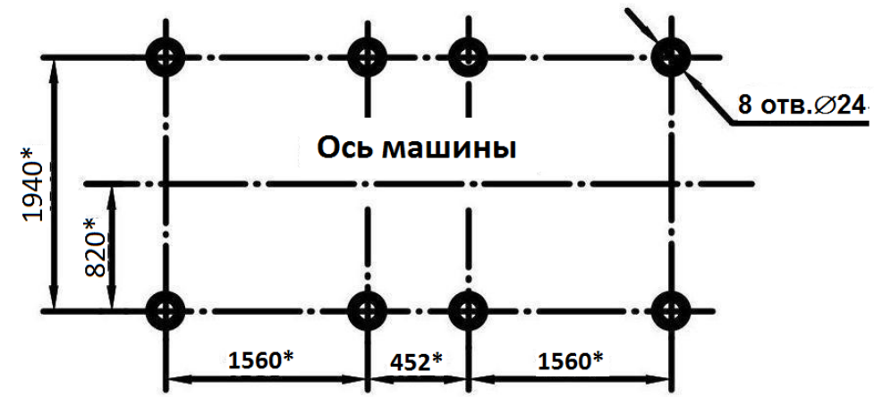
План расположения отверстий под фундаментные болты машины
