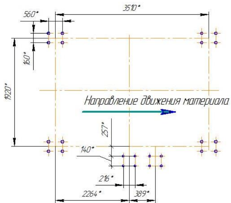
План расположения отверстий под фундаментные болты
