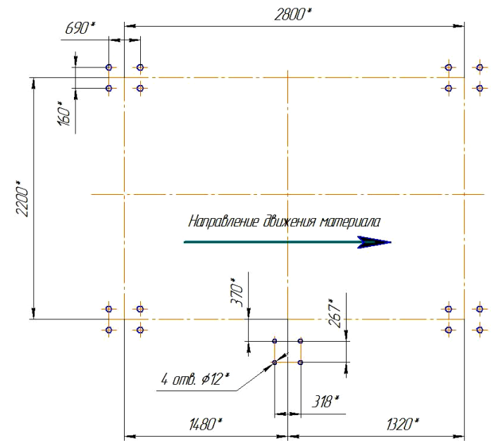
План расположения отверстий под фундаментные болты
